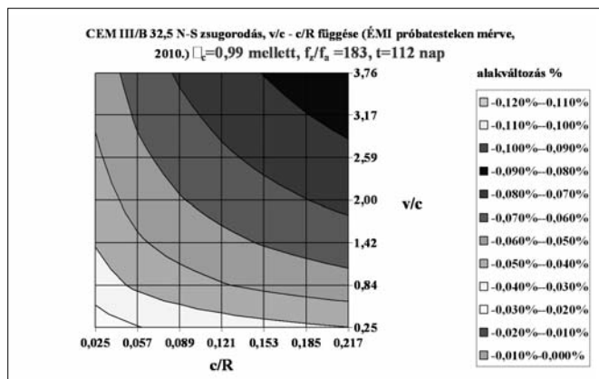
19. ábra CEM III/B 32,5 N-S cementtel készült keverékek v/c - c/R - \chi_c -alapú alakváltozás-becslő nomogramja t=112 napos korban, \chi_c=0,99 és f_z/f_a=183 (tisztá cementes péppor, közepes homoktartalmú adalékanyag) esetén
