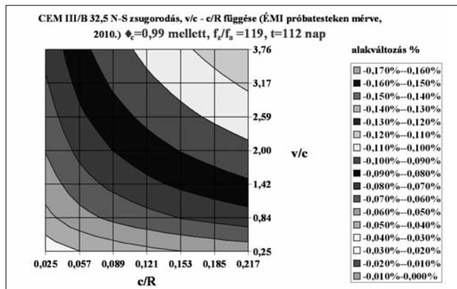
21. ábra CEM III/B 32,5 N-S cementtel készült keverékek v/c - c/R - \chi_c -alapú alakváltozás-becslő nomogramja t=112 napos korban, \chi_c=0,99 és f_z/f_a=119 (tisztá cementes péppor, homokdús adalékanyag) esetén
