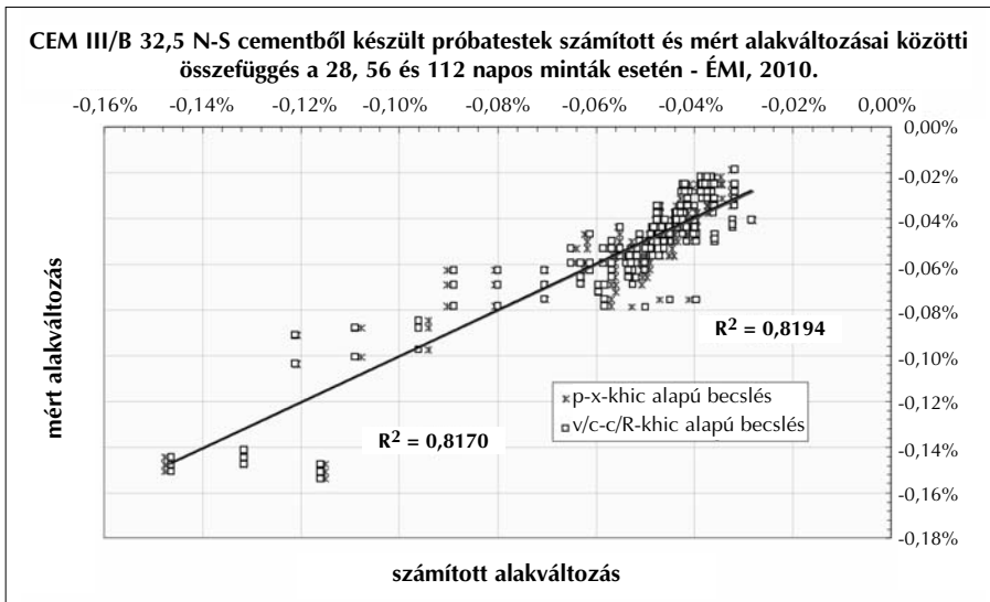
17. ábra A CEM III/B 32,5 N-S cementből készült próbatetek 28, 56 és 112 napos alakváltozásainak (35) illetve (36) képletekből becsült értékei és a ténylegesen mért értékek között, az ÉMI 2010. évi kérésletei során
