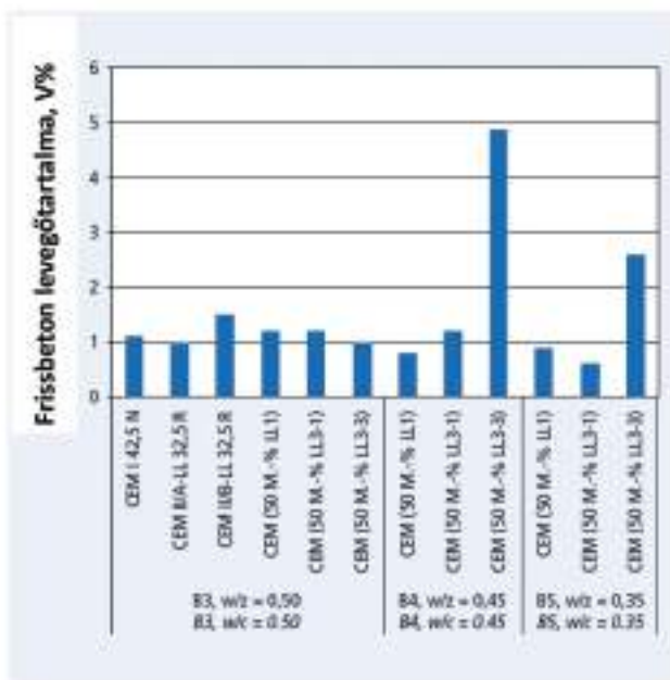
12. ábra: Üzemi cementekből és 50m/m% mészkőtartalmú kísérleti cementekből készített betonok nyomószilárdsága és levegőtartalma [12]
