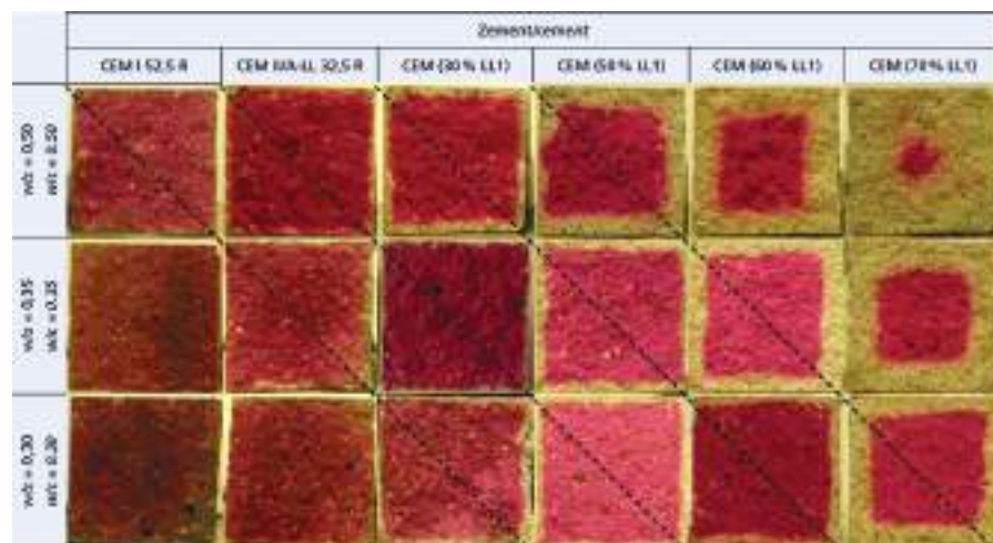
15. ábra: Üzemi cementekből és mészkőtartalmú kísérleti cementekből készített különböző víz/cement tényezőjű (w/z, ill. w/c) habarcs próbatestek karbonátosodása (-----ekvivalencia vonalak) [12] Impact of ENV 197 on Concrete Construction, pp.
