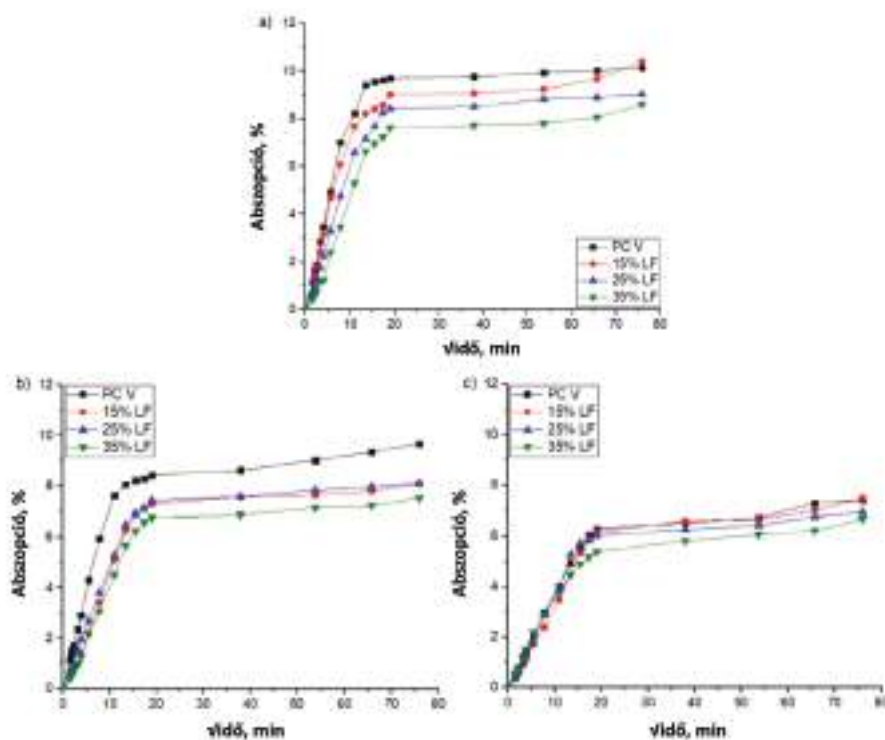
10. ábra: A portlandcement (PC V) kapillaris vízfelszívásának változása a mészkőtartalom (LF) és a víz/cement tényező ( a=0,58 ; b=0,50 ; c=0,42 ) függvényében [11]
