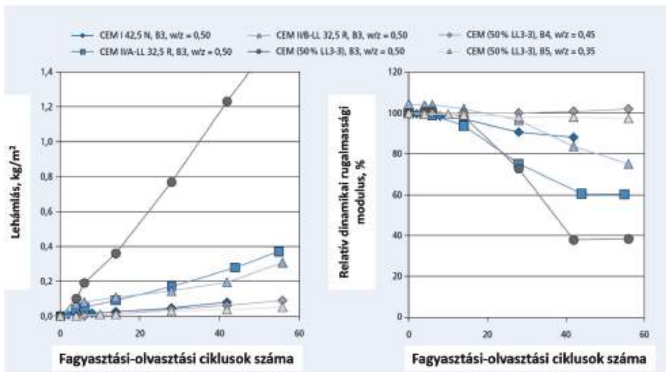
14. ábra: Üzemi cementekből és 50m/m% mészkőtartalmú (LL3-3) kísérleti cementekből készített betonok fagyállósága [12]
