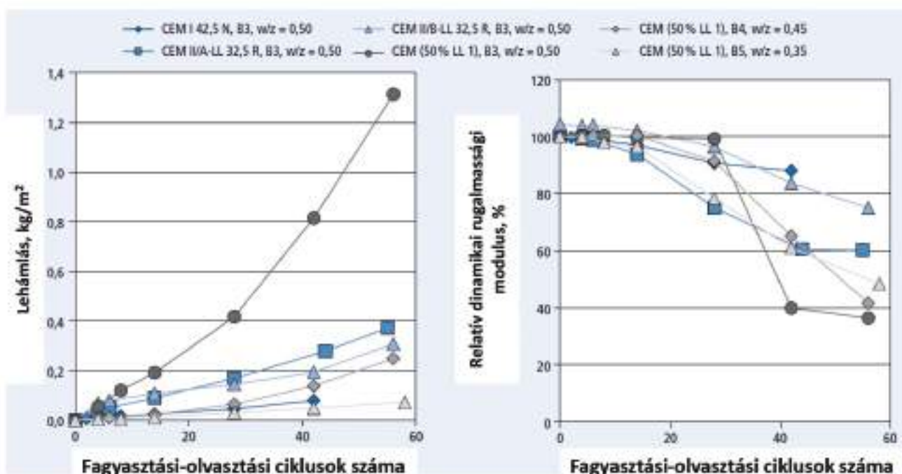
13. ábra: Üzemi cementekből és 50m/m% mészkőtartalmú (LL1) kísérleti cementekből készített betonok fagyállósága [12]
