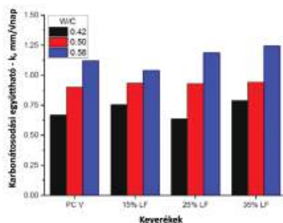
11. ábra: A portlandcement (PC V) karbonátosodási együtthatójának változása a mészkőtartalom (LF) és a víz/cement tényező ( w/c ) függvényében [11]
