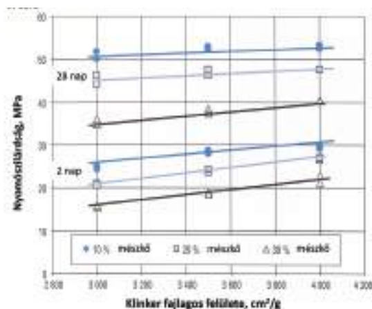
9. ábra: A cement nyomószilárdságának változása a mészkőtartalom és az őrési finomság (különőrlés) függvényében [10]
