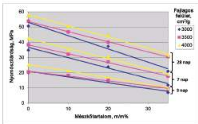
8. ábra: A cement nyomószilárdságának változása a mészkőtartalom és az őrési finomság (együttőrlés) függvényében
