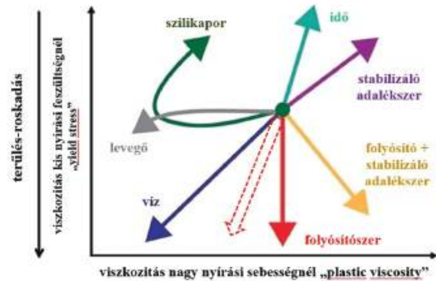
10. ábra Pépösszetevők hatása a reológiai jellemzőkre [35]
