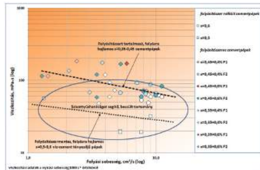
11. ábra Cementpékek folyási sebessége és viszkozitása nagy nyírási sebességnél
