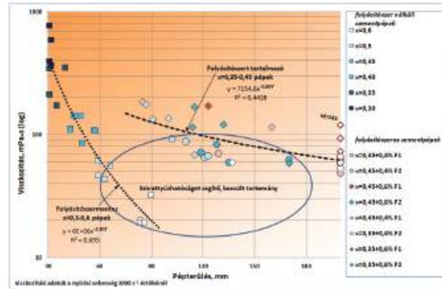
9. ábra Cementpépek területe és viszkozitása nagy nyírási sebességnél
