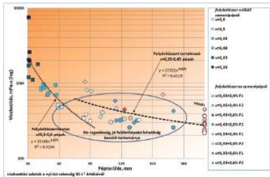
8. ábra Cementpépek területe és viszkozitása kis nyírási sebességnél
