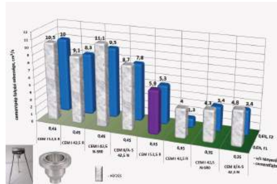
4. ábra: Cementpépek folyási sebessége és vérzési hajlama v/c=0,35 ; 0,45 és 0,6\text{ m\%} (magnövelt) F1 és F2 folyósítószer adagolása mellett
