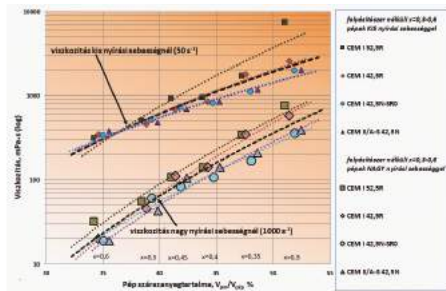
5. ábra: Folyósítószermentes cementpépek szárazanyagtartalma (v/c) és viszkozitása kis és nagy nyírási sebesség esetén
