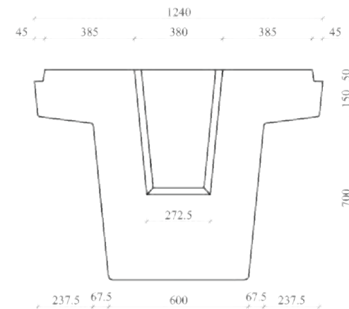
2. ábra A tartóvég vázlata (mértékegység: mm) és fényképfelvétele
