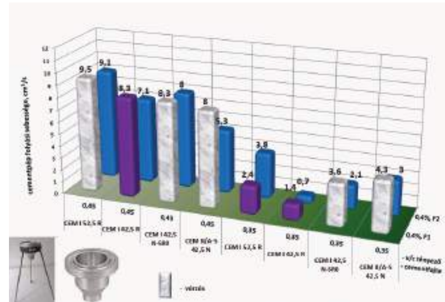
3. ábra: Cementpépek folyási sebessége és vérzési hajlama v/c=0,35 ; 0,45 és 0,6\text{ m\%} F1 és F2 folyósítószer adagolása mellett
