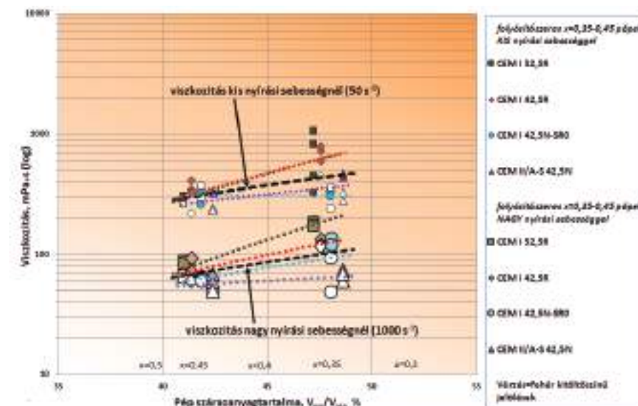
6. ábra: Folyósítószeres cementpépek szárazanyag-tartalma (v/c) és viszkozitása kis és nagy nyírási sebesség esetén
