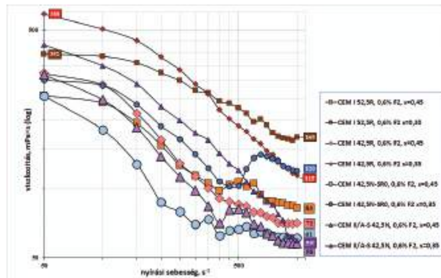
7. ábra: Folyósítószeres cementpépek viszkozitása és nyírási sebessége
