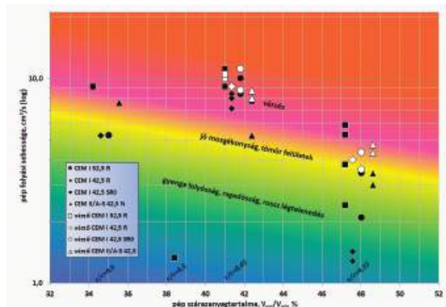
2. ábra: Mozgékony pépek folyási sebessége és a betonkeverék ebből becsült viselkedése
