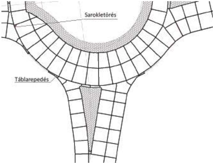
3. kép - Repedéstérkép a táblakiosztási terven (készítette: Dr. Bencze Zsolt)
