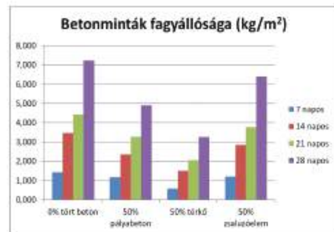
6-7. ábra - Friss- és megszilárdult beton vizsgálati eredmények
