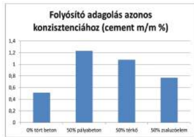
5. ábra - Azonos területi osztály eléréséhez szükséges folyósítószerigény
