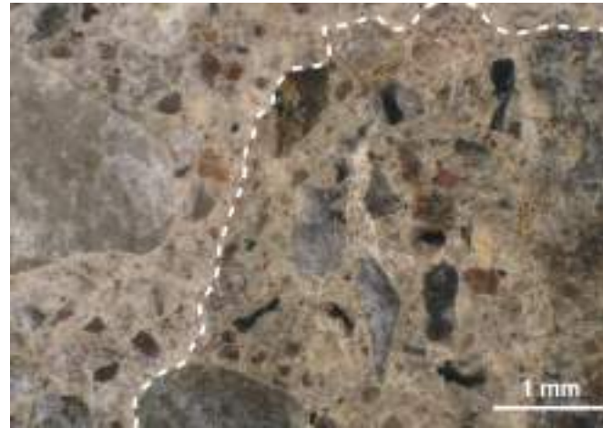
3 kép: Tört betonnal (zsaluzóelem) készült betonok mikroszkópi felvételei
