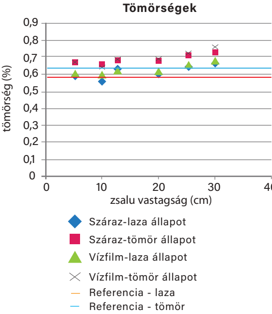
2. grafikon 4-8 frakció halmaztömörégeinek összehasonlítása
