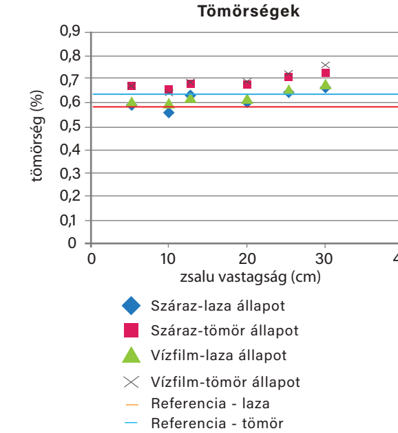
3. grafikon 8-16 frakció halmaztömörégeinek összehasonlítása
