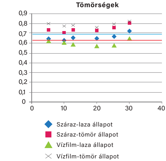
1. grafikon 0-4 frakció halmaztömörégeinek összehasonlítása
