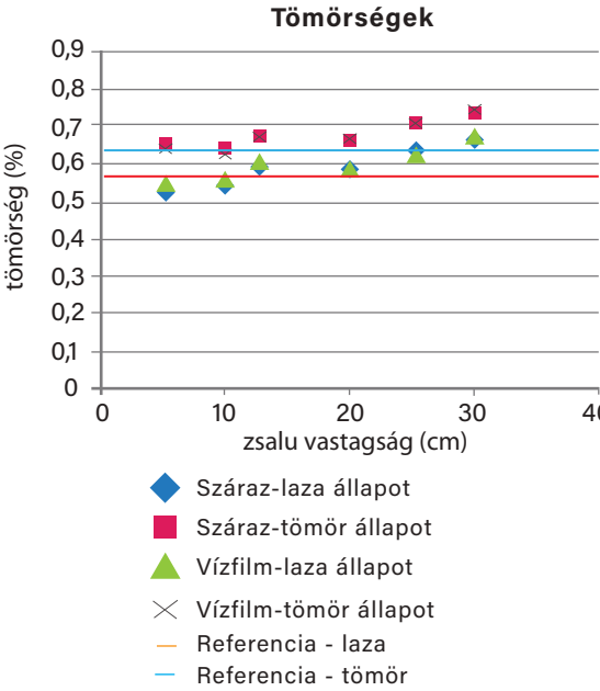
4. grafikon 16-32 frakció halmaztömörégeinek összehasonlítása
