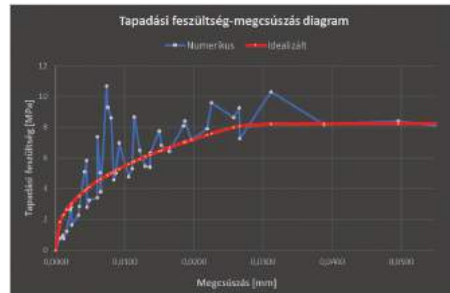
4. ábra: Tapadási feszültség-megcsúszás diagram bordázott betonacél esetén
