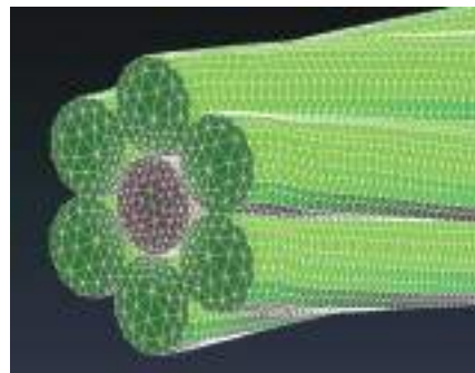
2. ábra: A héteres acélpászma végeelemes hálója
