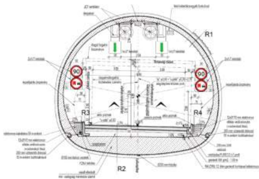
Az alagút tervezett mintaszelvénye
