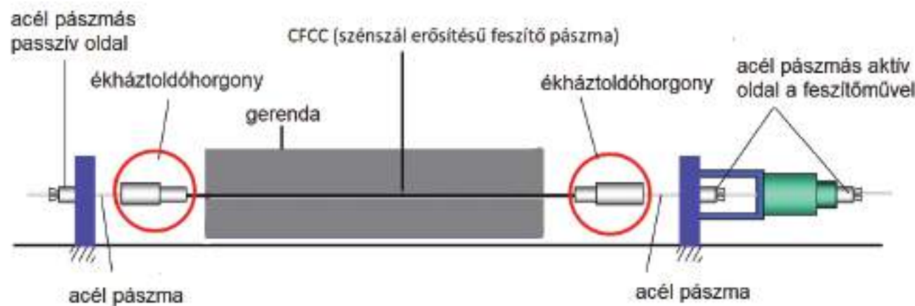
1. ábra Elvi rajz CFCC
