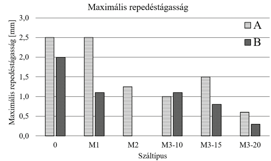
5. ábra. Maximális repedésméretek a különböző vizsgálatoknál
