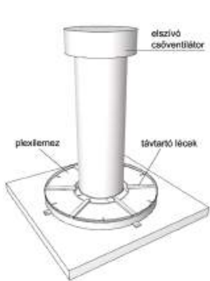
2. ábra a) RF által ajánlott szárító elrendezés [3] b) Fenyvesi [2] által ajánlott szárító elrendezés
