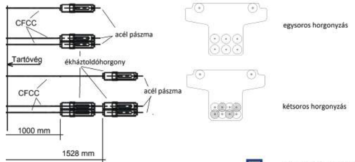
3. ábra Variációk CFCC összekötésére
