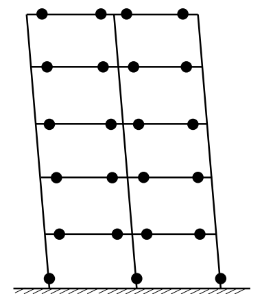
4. ábra Tervezett képlékeny csuklók helye vasbeton váz esetén
