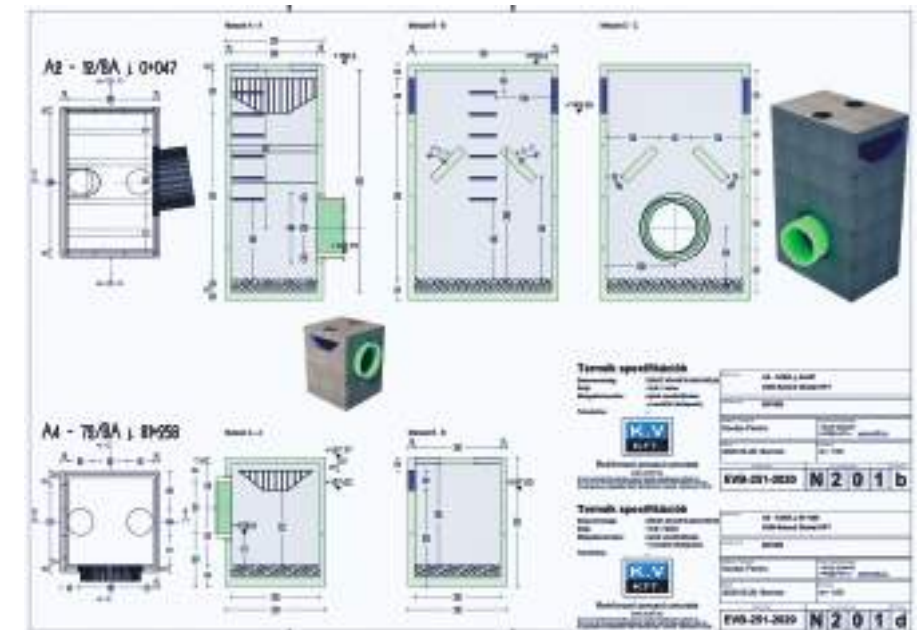
Egyedi vasbeton akna átdolgozott gyártmányterve
