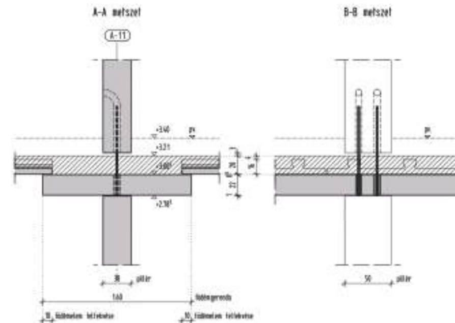
3. kép: Az alsóbb szint pilléreiből kiálló betonacél tüskék átmennék a födémre és fogadják a következő szint pilléreit
