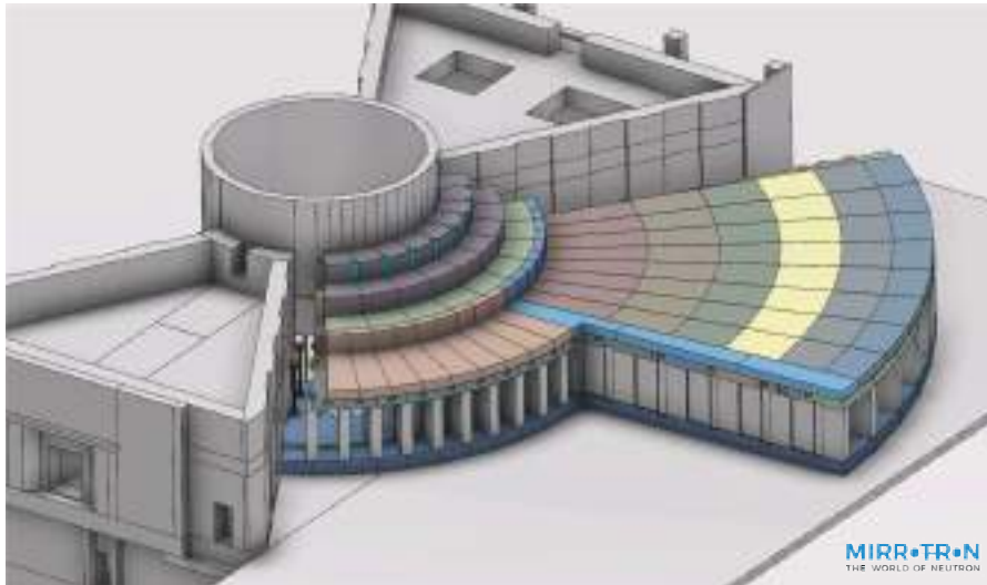
1. kép A bunker 3D-s modellje a nehézbeton falakkal és födémekkel (forrás: https://europeanspallationsource.se )
