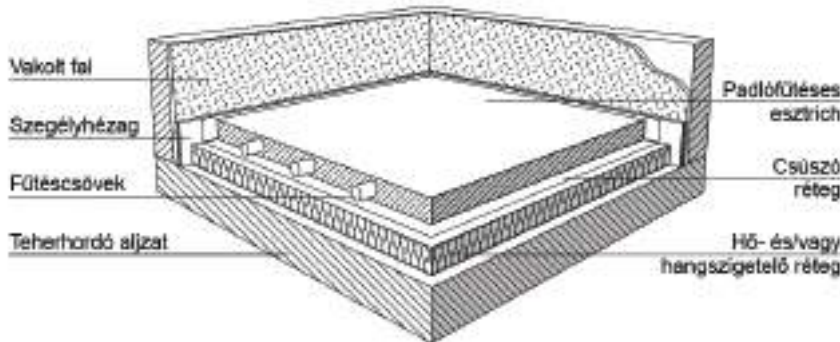
2. ábra: Padlófűtési esztrich (forrás: Padló MI 01:2015)
