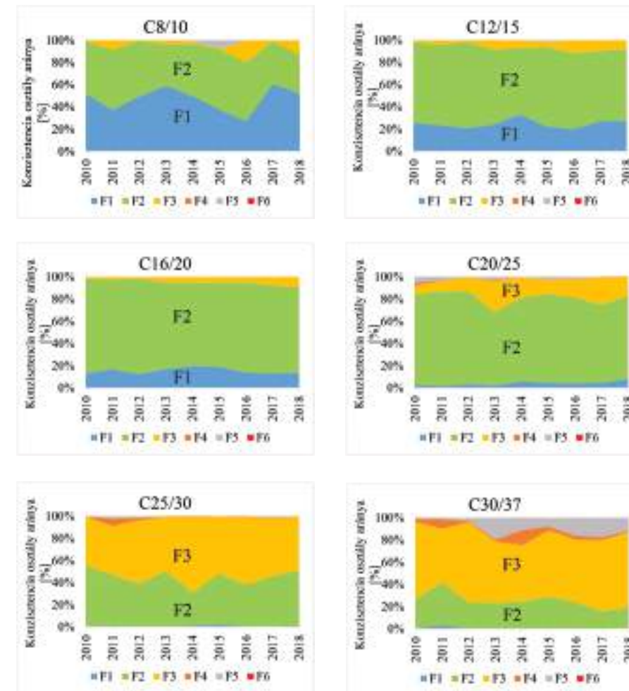
1. ábra: Konzisztenciaosztályok alkalmazásának aránya a nyomószilárdsági osztály függvényében az MSZ 4798 szabvány szerinti transzportbetonok esetén a Duna-Dráva Cement Kft. betonüzemeiben
